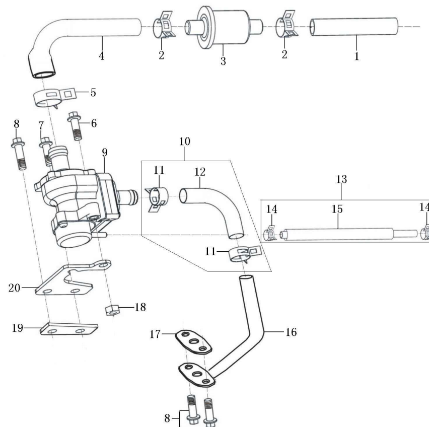
废气再循环系统 EXHAUST GAS RECIRCULATION SYSTEM
