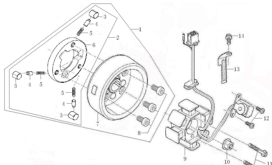
磁电机总成 MAGNETO COMP
