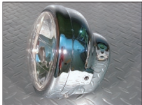
商品名 モニキーゴリラマルチリフレクターヘッドライト 税込価格 4,900円 商品説明 ダイヤモンドカットのリフレクター反射板を用い、照度が各角度にアップ、対向車からの認知度アップ 商品ID NO1002
