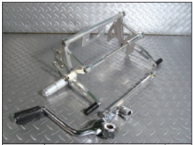
商品名 モンキーアルミ製バックステップディスクブレーキ用 税込価格 15,000円 商品説明 公道走行を前提にライディングポジションを考え設計、シフター加工必要 商品ID NO965
