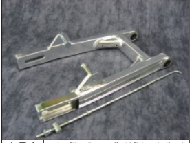
商品名 モンキーゴリラ+5cmロングアルミ製リアスイングアーム 税込価格 6,000円 商品説明 ホンダ純正リアスイングアームの形状のまま+5cmロングに変更可能なスイングアーム 商品ID NO1158
