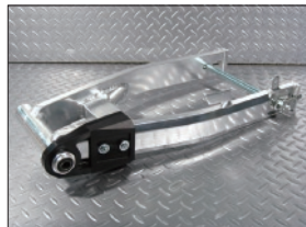
商品名 エイブ50100リアスイングアームアルミ製 税込価格 8,900円 商品説明 モンキーやゴリラを使用することで、強度アップと剛性が高く、ハイパワーなエンジンにも最適 商品ID NO628
