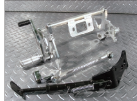
商品名 モンキーバックステップ専用サイドスタンド 税込価格 17,000円 商品説明 モンキーゴリラバックステップ [アルミ製 CNC] 専用可変サイドスタンドセット 商品ID NO879
