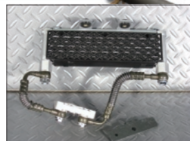
商品名 超激冷激熱大!モンキー大型オイルクーラーセット 税込価格 8,500円 商品説明 モンキー、ゴリラなどに最適な大型オイルクーラー、空冷有効サイズはH60mmxL210mm 商品ID NO887
