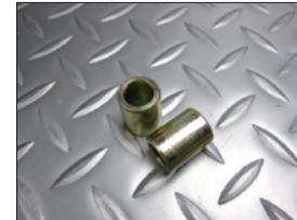
商品名 リアショック M10 カラー左右セット 税込価格 400 円 商品説明 仕様内径 10mm、外径 16mm、幅 21mm 商品ID NO1334
