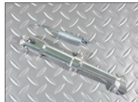
商品名 モンキーCNCアルミ製8インチサイドスタンド 税込価格 2,800円 商品説明 有効長約200mm、アルミ製 CNC スタンド、購入前に長さをご確認ください 商品ID NO908
