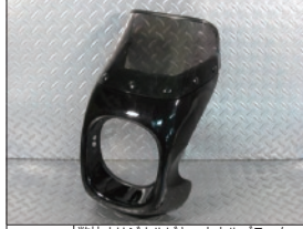
商品名 弊社オリジナルビキニカウルブラック 税込価格 4,900円 商品説明 高さ380mm、横幅200mm、突き出し140mm(平置き状態で測定)、モンキー、エイブ取り付け可 商品ID NO295
