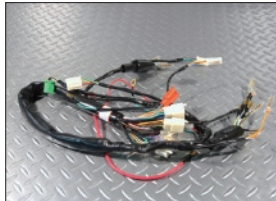
商品名 モンキー 12V メインハーネス 税込価格 2,800 円 商品説明 一括交換を目的とした12Vハーネスセットをお探しの方はNO28がおススメ 商品ID NO814
