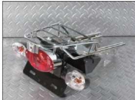
商品名 モニキーリアキャリア純正仕様12Vウィンカー 税込価格 6,800円 商品説明 ウィンカー2ヶ付テールランプ、工具ボックスが付属、ホンダモトキーモトキースタイルバイクにオススメ 商品ID NO842
