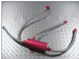
商品名 オイルキャッチタンクレッド 税込価格 4,200円 商品説明 タンク長さ40mm、タンク直径55mm、ステンレスメッシュホース仕様 商品ID NO333
