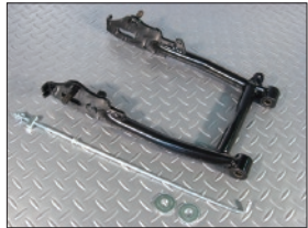
商品名 モンキーゴリラ+5cmロング黒リアスイングアーム 税込価格 5,000円 商品説明 ホンダ純正リアスイングアームの形状のまま+5cmロングに変更可能なスイングアーム 商品ID NO1009
