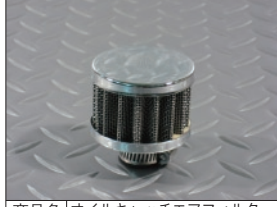
商品名 オイルキャッチエアフィルター 税込価格 600円 商品説明 オイルキャッチタンクエアフィルター、排圧ホースに取り付け、M8 ホース適合 商品ID NO355
