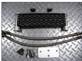
商品名 160ccエンジン専用ホース付きオイルクーラーセット 税込価格 7,200円 商品説明 160cc エンジン専用のオイルクーラー、オイルクーラー側M12x 取り出し口側M8 商品ID NO1029
